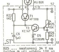
DESKA STABILIZÁTORU (samostatná deska „ST“)
