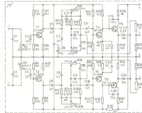
TÓNŮV KOREKCE (samostatná deska „TK“)
