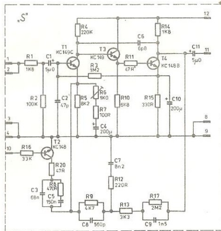
SNÍMÁČÍ ZESILOVAČ (modul „S“ v základní desce „ZD“ - použit 2x)
