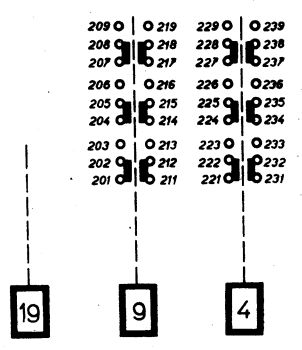
PŘEPÍNAČ RYCHLOSTÍ
