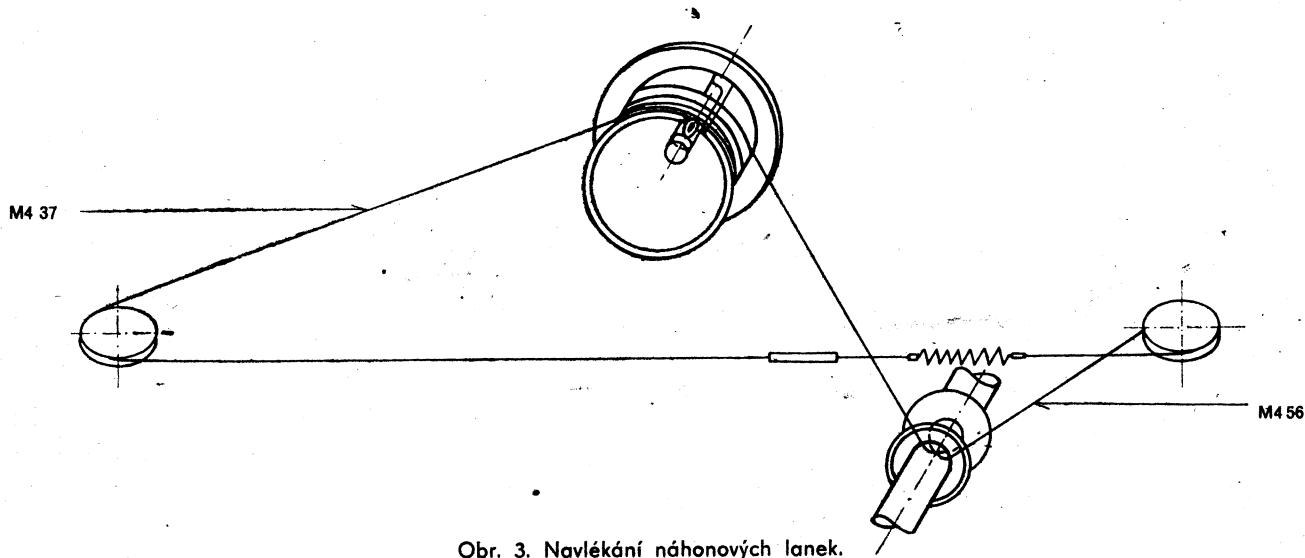
Obr. 3. Navlékání náhonových lanek.
