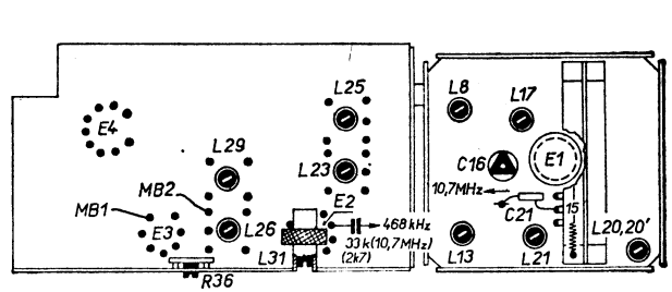
Sladovací prvky pod šasi
