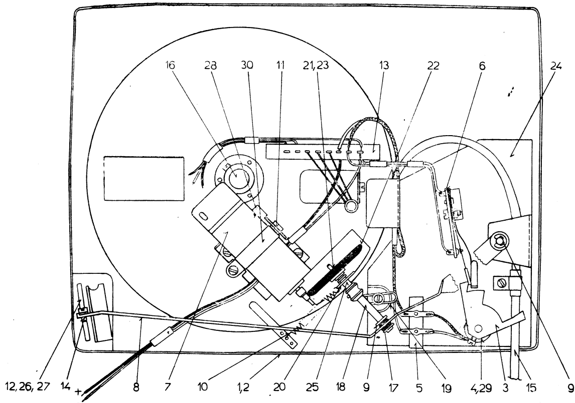
Obr. 3. Chassis gramofonu
