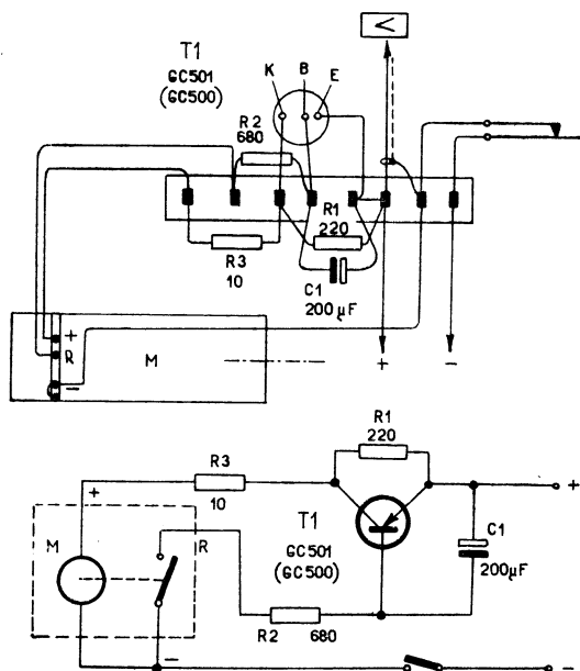
Obr. 2. Zapojení tranzistorové regulace
