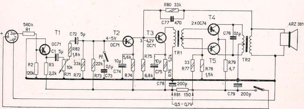
Obr. 5. Schéma zesilovače
